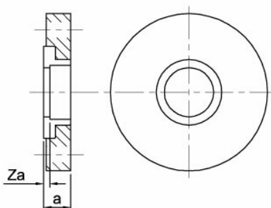
N1FMGI Flange
